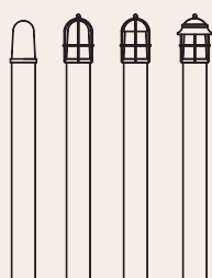
D 11cm H 115cm 1x75W E27 IP44 1x23W E27 IP44
