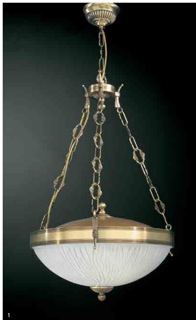
1. L 5610/3 bronzio arte, vetro bianco ↑ 72 ↔ 42 3 x max60W E27
